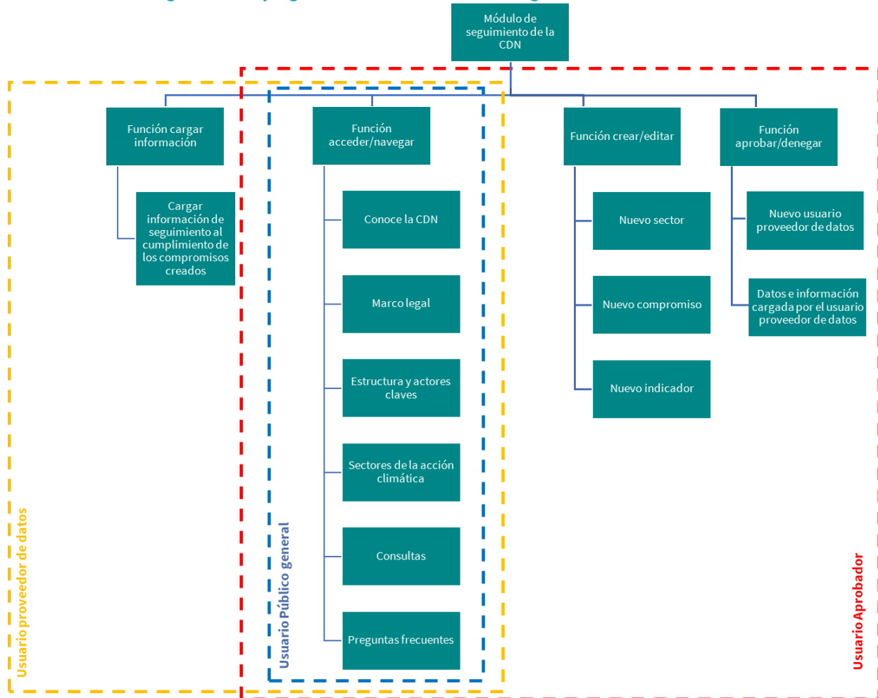
Figura 3: Flujo general del Módulo de Seguimiento de la CDN
